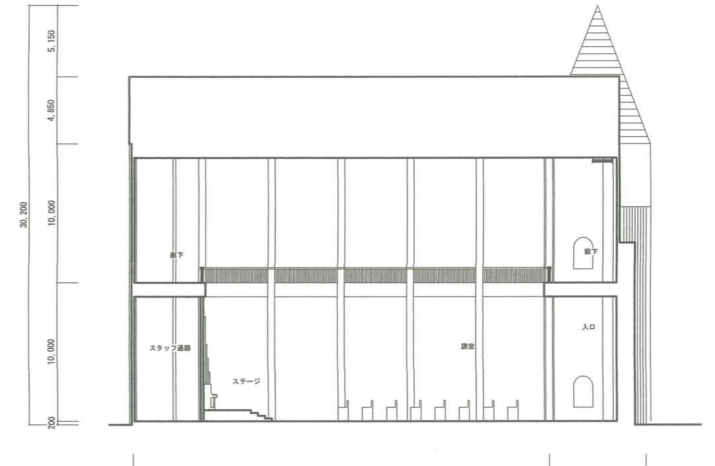
断面図 1/250
