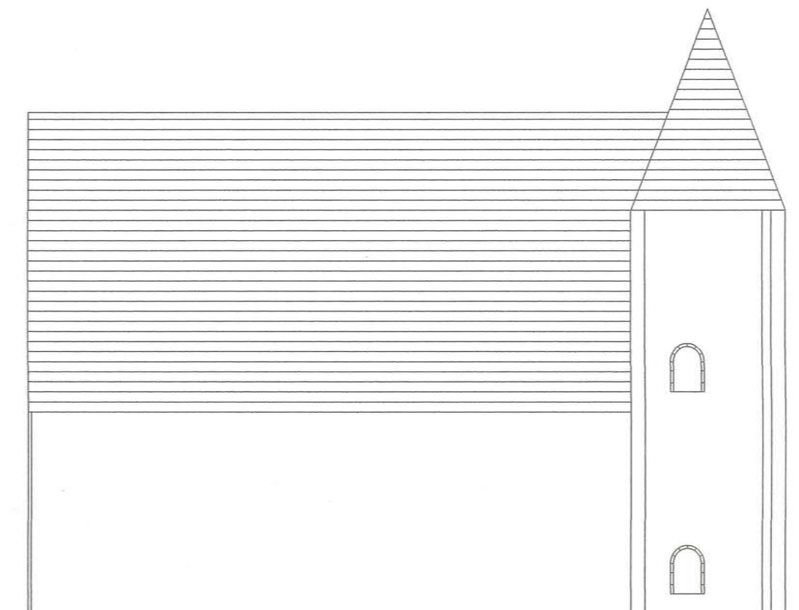
北立面図 1/200
