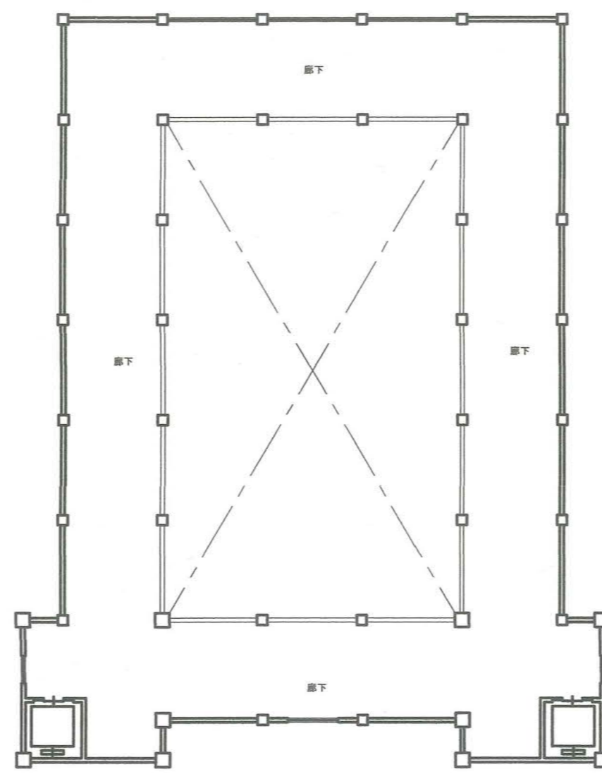
二階平面図 1/250
