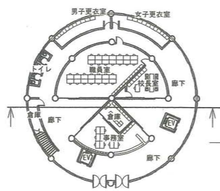
一階平面図 1/500
