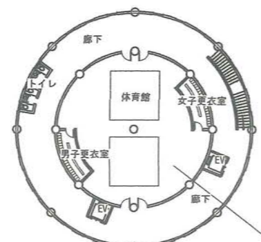
四階平面図 1/500
