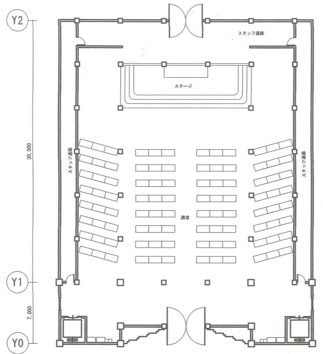
一階平面図 1/250
