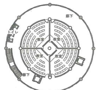
六階平面図 1/500
