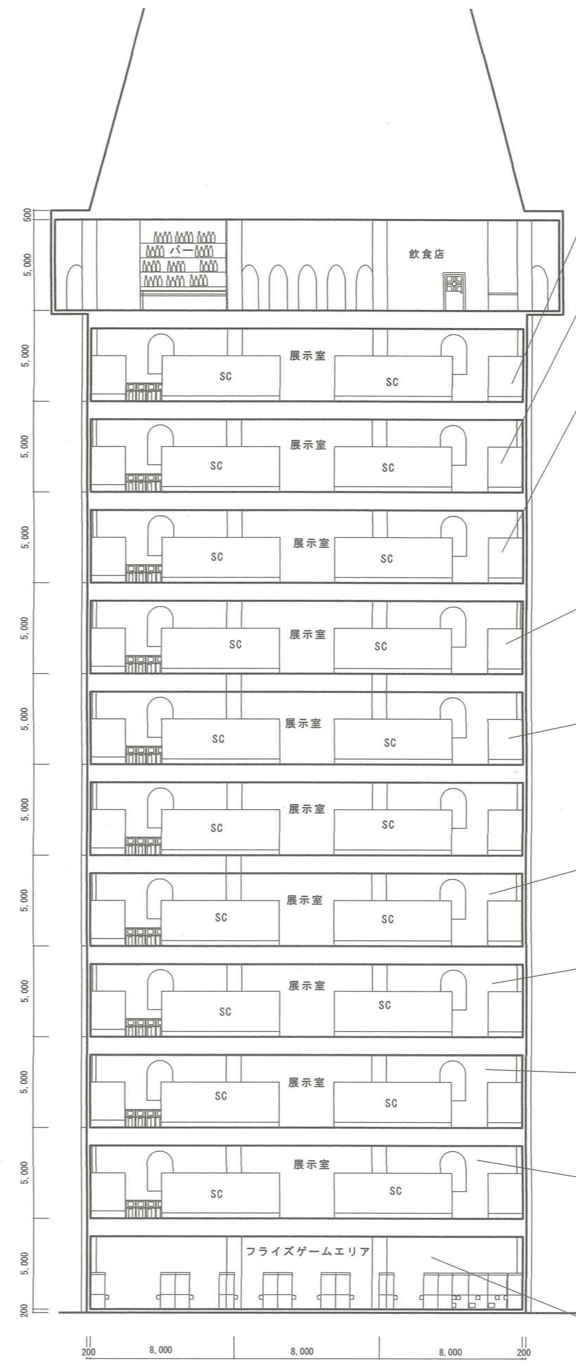
断面図 1/200
