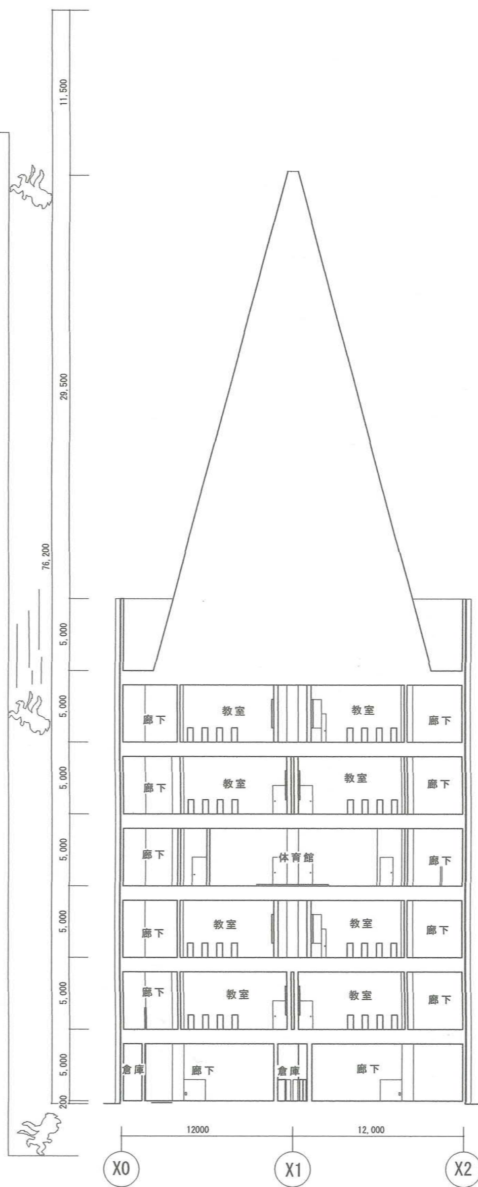
断面図 1/250
