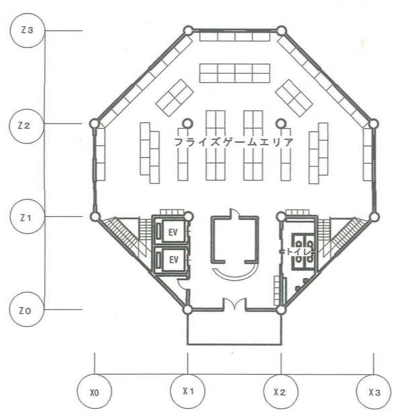
一階平面図 1/300
