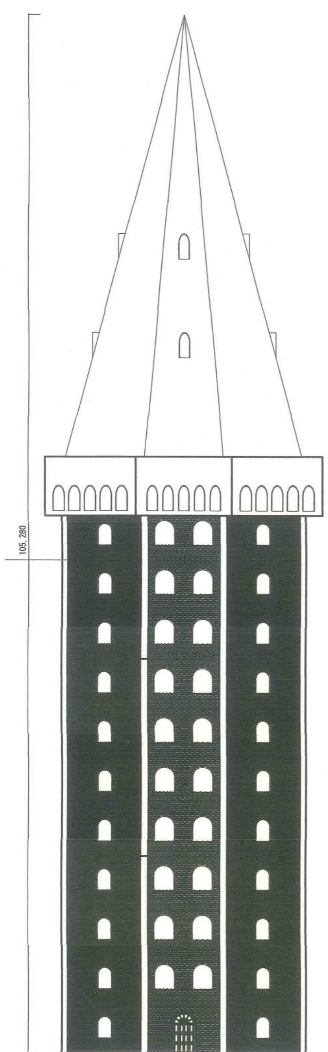
立面図 1/300
