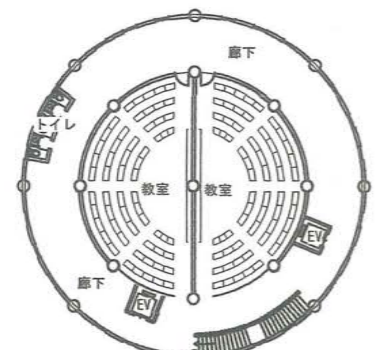
五階平面図 1/500
